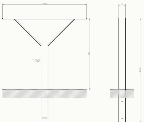
Ausführung P1 zum Einbetonieren
