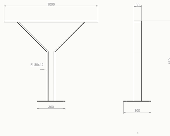
Ausführung P1 zum Aufdübeln
